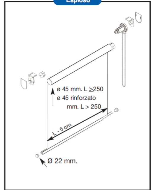
Esploso
